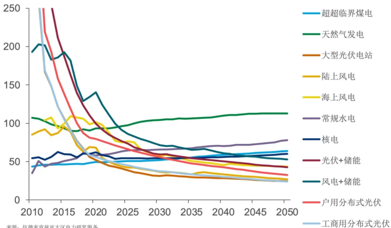
中国各电源平准化发电成本 (US$/MWh)
